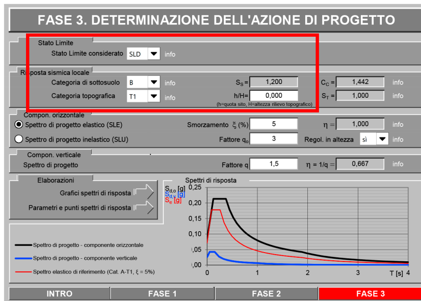
Fig. 39 Definizione degli spettri di risposta: fase 3
